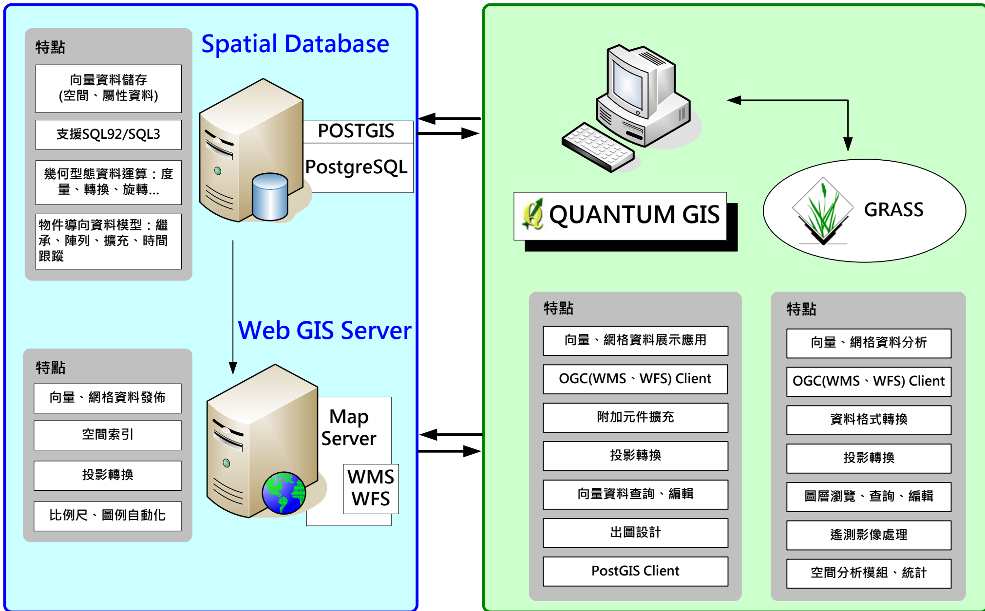
QUANTUM GIS與周邊相關軟體關係圖
